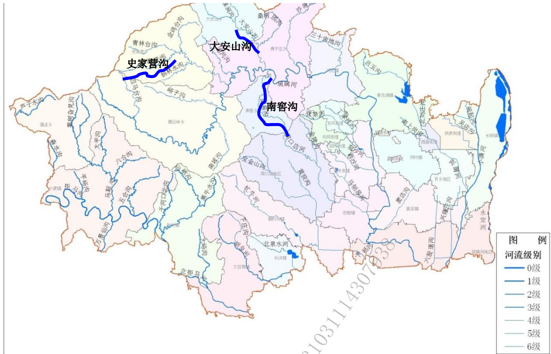
图 1.2-1 房山区主要河流水系图
